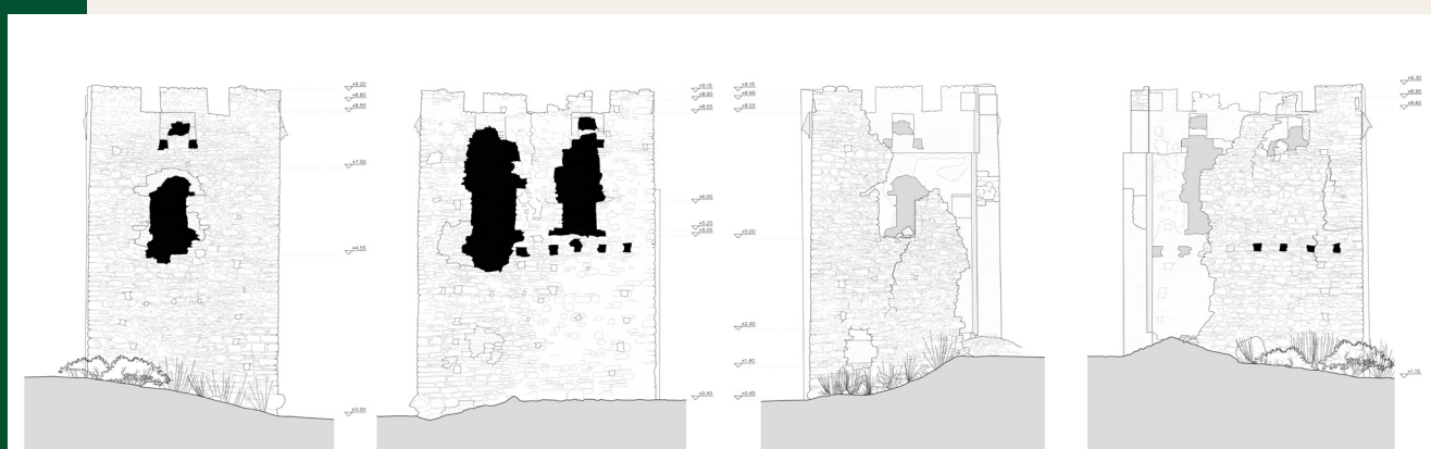
3. Σχεδιαστική αποτύπωση της υφιστάμενης κατάστασης του Πύργου (σχέδιο Κ. Δημητρούλιας). Plan of the existing situation of all four sides of the tower (plan by K. Dimitroulias).
